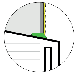
Anschluss unten
